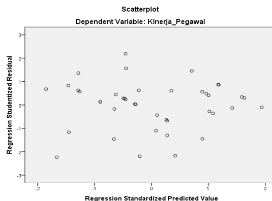
Gambar 2. Grafik Heteroskedastisitas
